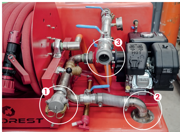
1- Succión externa | 2- Succión interna | 3- Boca de expulsión
